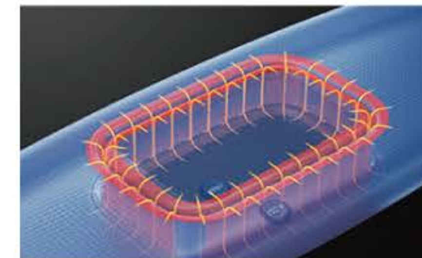
60Lの浮力確保
